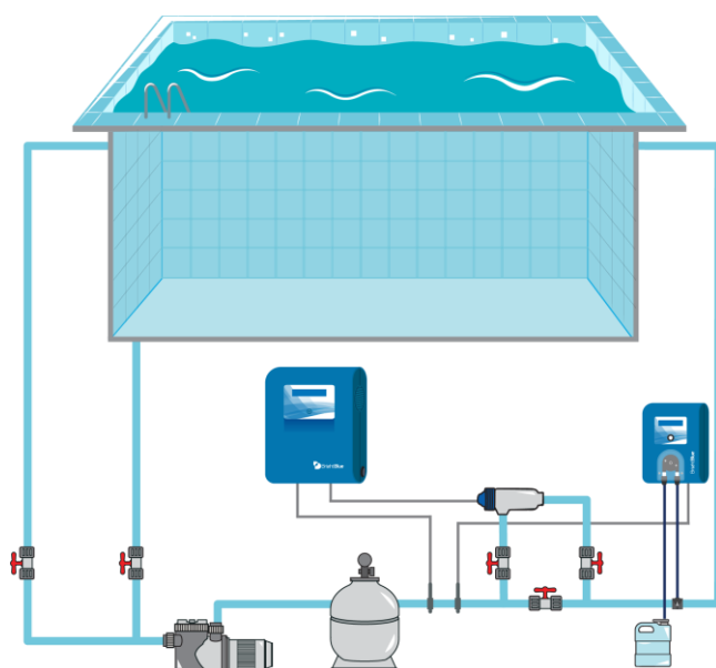
Figura 2B- Representação Hidráulica do Sistema SENSUS versão bomba injectora
