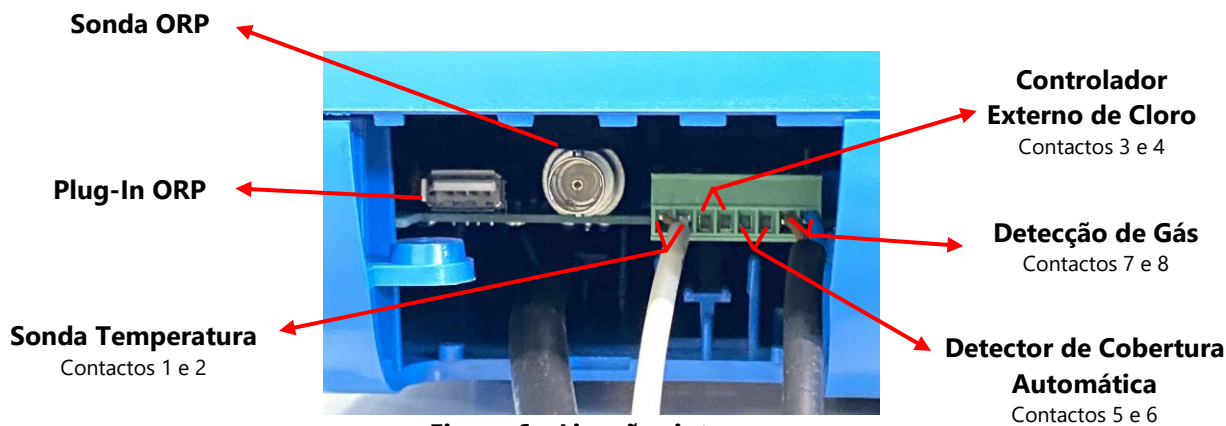
Figura 6 – Ligações internas
