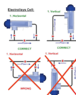
Figura 3- Posição da Célula de Electrólise
