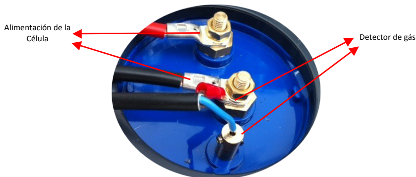
Figura 5 – Terminales de Conexión en la Celda
