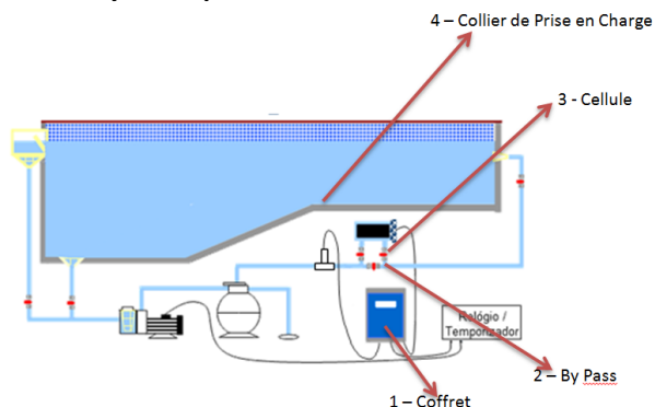
Fig 4- Système hydraulique
