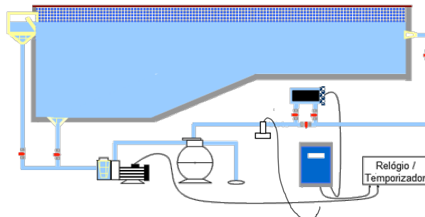
Figura 2- Representación Hidráulica del Sistema
