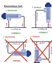
Fig 3 – Position de la cellule
