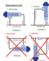
Figura 3- Posición de Celda de Electrolisis
