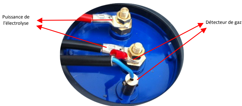
Fig 5 – Bornes de connexion de cellule d'électrolyse
