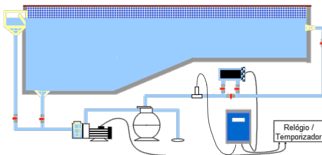
Figura 1- Representação Hidráulica do Sistema
