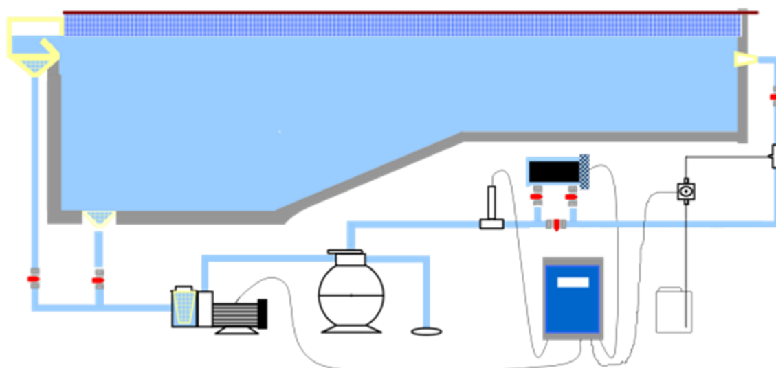
Figura 2- Representação Hidráulica do Sistema
